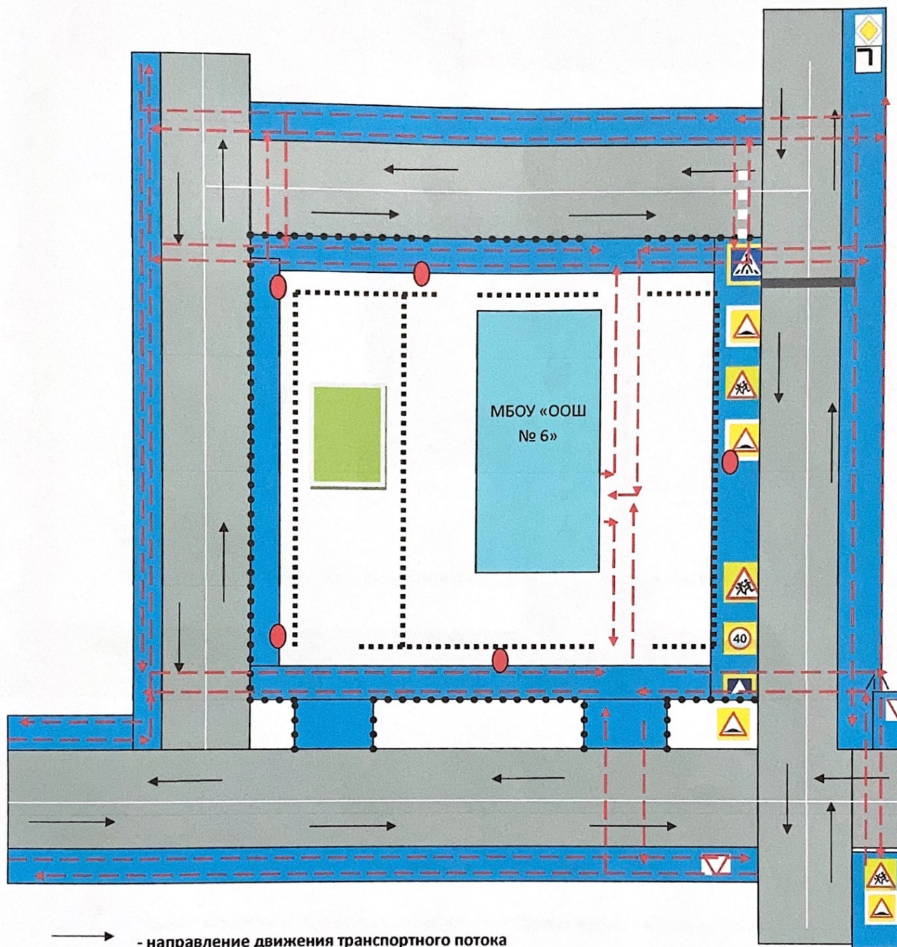
2. Схема организации дорожного движения в непосредственной близости от образовательной организации с размещением соответствующих технических средств организации дорожного движения, маршрутов движения детей и расположения парковочных мест.
